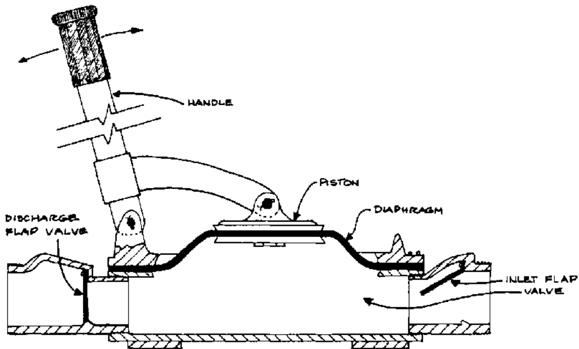
FIG. VII-9. DIAPHRAGM PUMP
